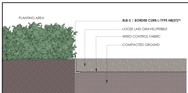
รูปตัดแสดงการติดตั้ง BL8-S | BORDER CURB L-TYPE H8 (ST) TM และโรยกรวด
