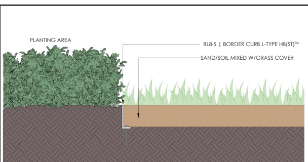
รูปตัดแสดงการติดตั้ง BL8-S | BORDER CURB L-TYPE H8 (ST) TM และปลูกหญ้า
