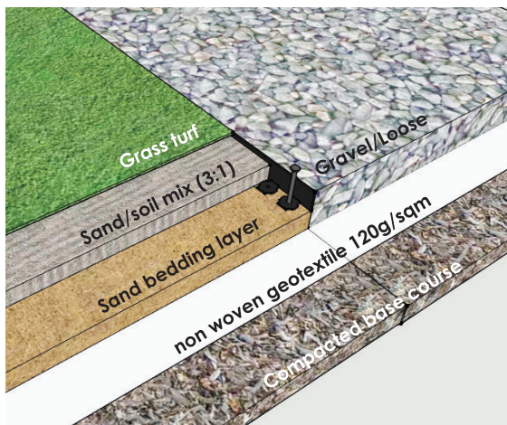
รูปตัดแสดงการติดตั้ง BL8-S | BORDER CURB L-TYPE H8(ST) TM
