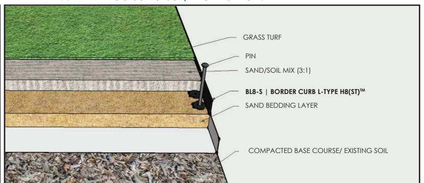
รูปแสดงการติดตั้ง BL8-S | BORDER CURB L-TYPE H8 (ST) TM และปลูกหญ้า
