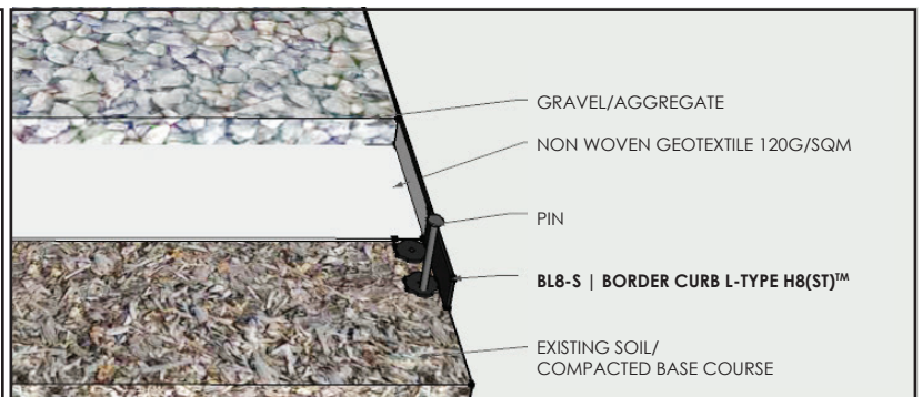
รูปแสดงการติดตั้ง BL8-S | BORDER CURB L-TYPE H8 (ST) TM และโรยกรวด
